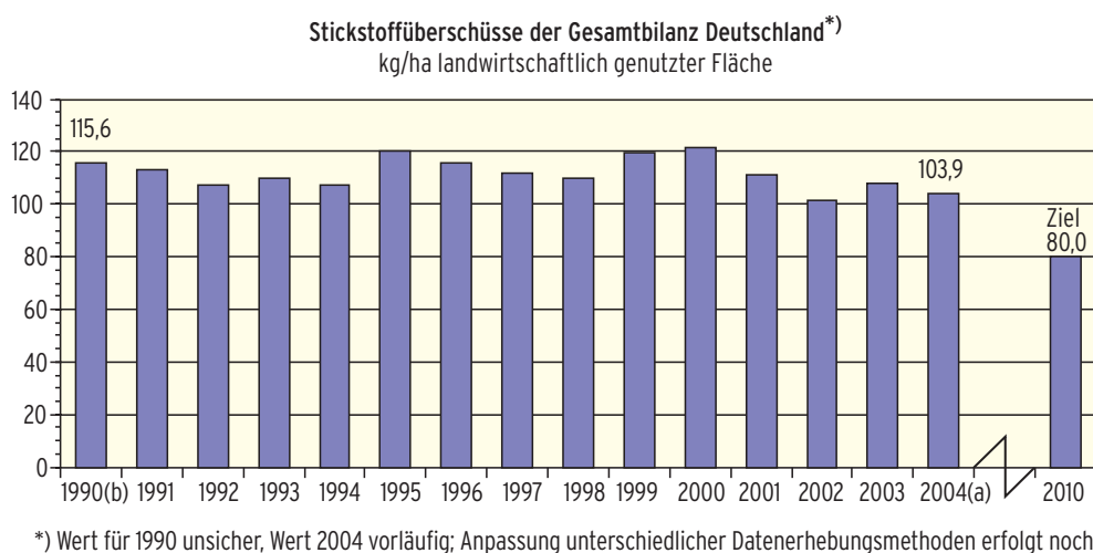
Abb. H 12: Stickstoffüberschüsse der Gesamtbilanz Deutschland*)
